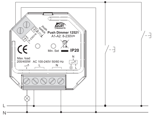
Ledningsdiagram
